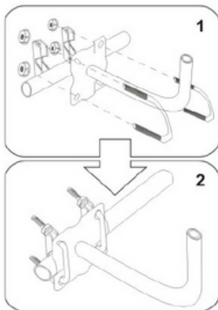
Soporte de barandilla
